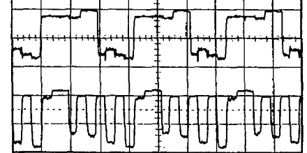
Q803 collector 100v p.p. Spitze- Spitze bei 20 \mu sec
