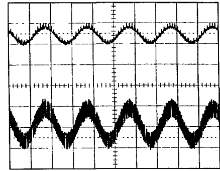
IC4051 pins 8/15 1v 2 p.p.Spitze- Spitze bei 0.5m sec
