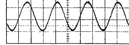
IC4450 pins 8/10 1v3 p.p.Spitze- Spitze bei 1m sec
