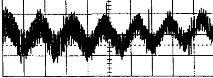
IC4201 pin 29 0.56v p.p.Spitze- Spitze bei 10m sec
