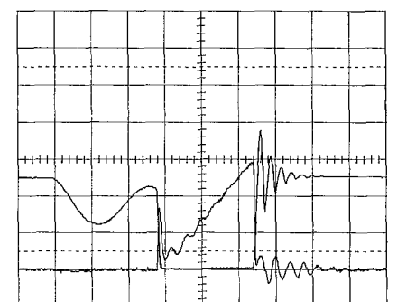
Sub PSU Q9002 VCE 720V p.p. Spitze- Spitze bei 2 \mu sec
