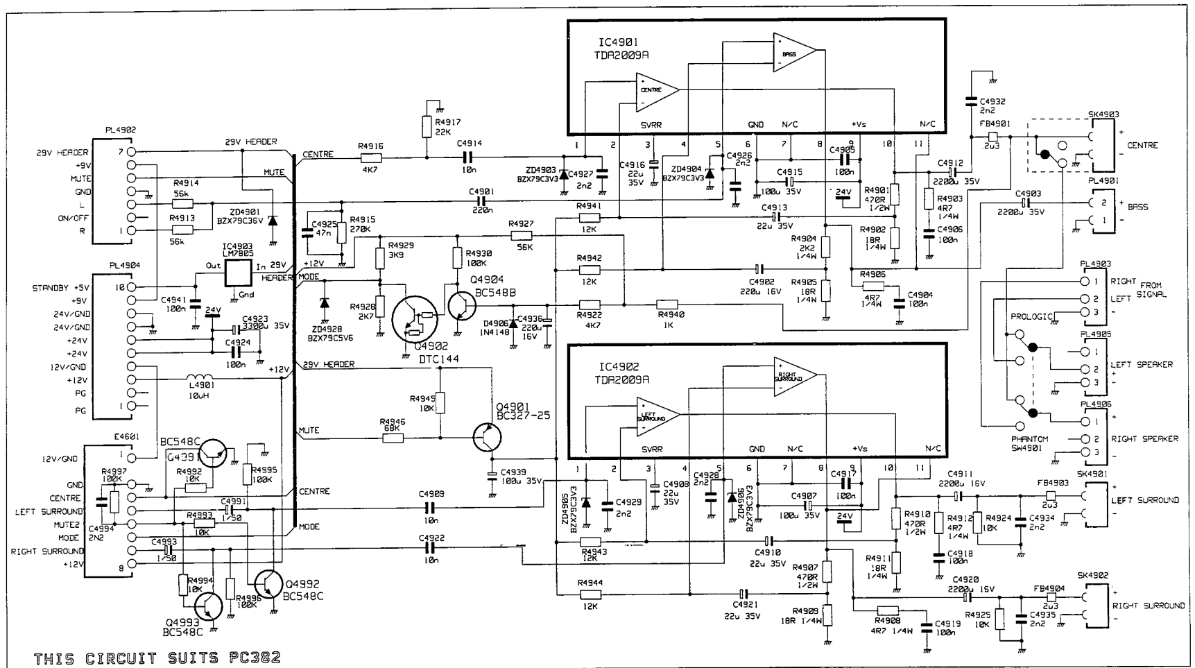
AUDIO SUB-AMP CIRCUIT AKUSTISCHE-VERSTÄRKERPLATINE
