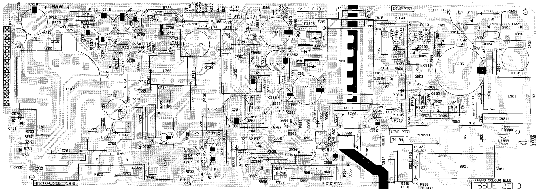
POWER SUPPLY AND DEFLECTION P.C.B. PRINT SIDE NETZTEIL UND ABLENKPLATINE, GEDRUCKTE SEITE
