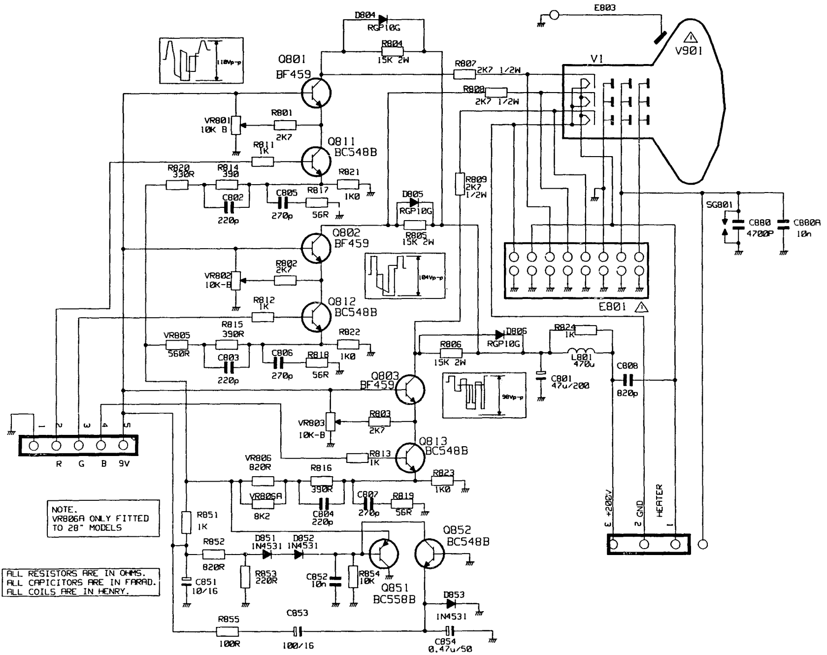
C.R.T. BASE CIRCUIT BILDROHREN-PLATINE
