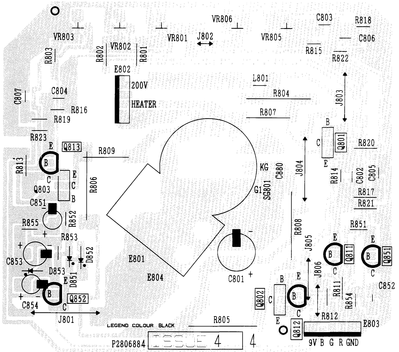
C.R.T. BASE P.C.B. PRINT SIDE BILDROHREN-PLATINE, GEDRUCKTE SEITE
