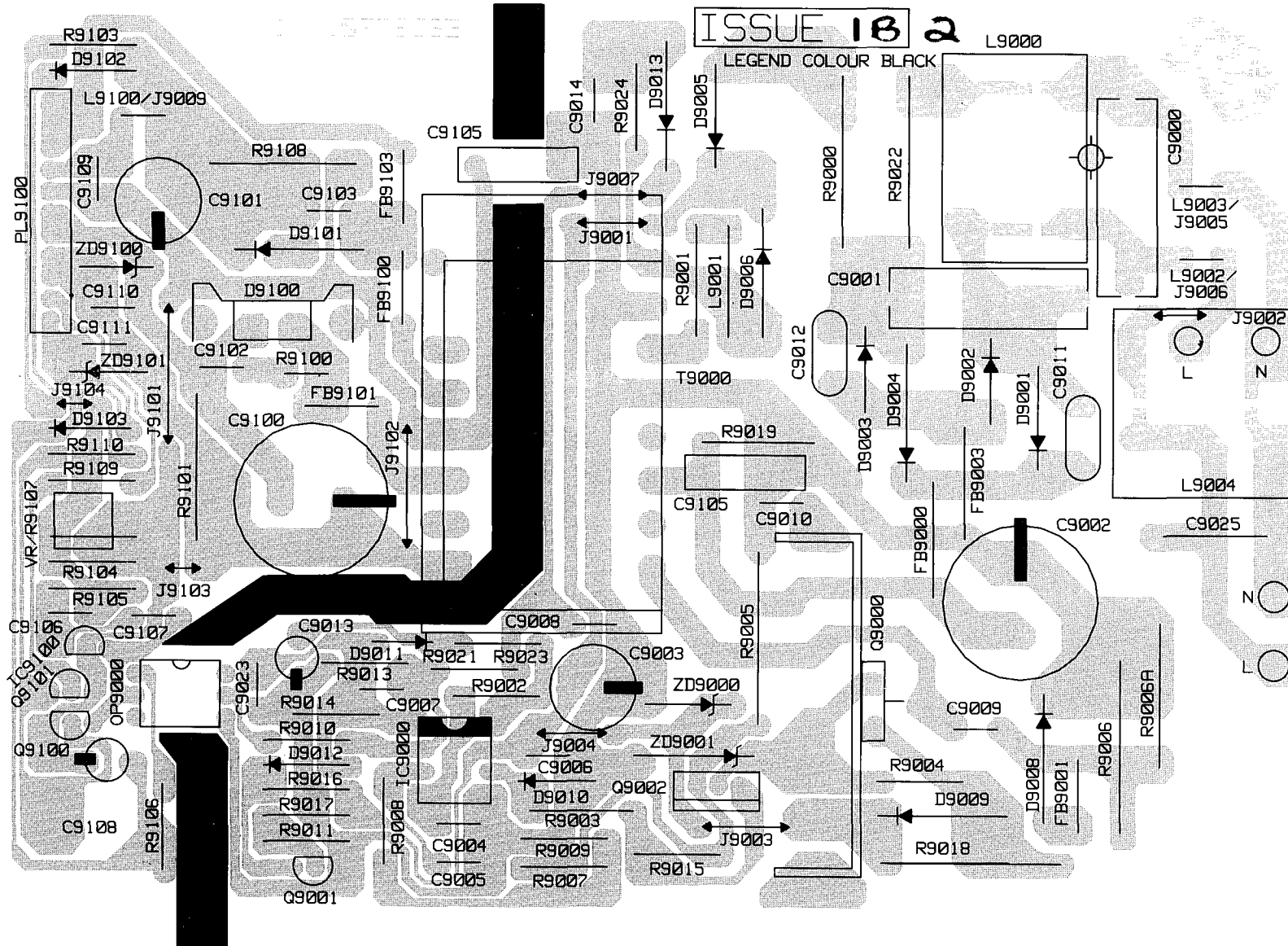
POWER SUPPLY SUB-PANEL P.C.B. PRINT SIDE STROMVERSORUNGSP-LATINE, GEDRUCKTE SEITE
