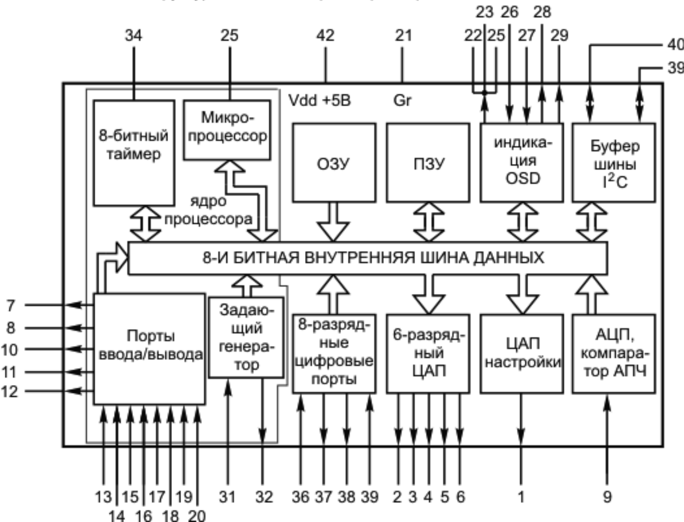
Структурная схема микроконтроллера INA84C64INS-168
