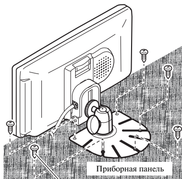
Винты-саморезы (3 x 12 мм)
