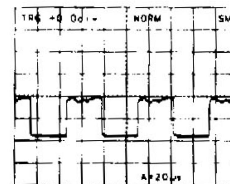
⑪ 4.5 Vp-p (H)
