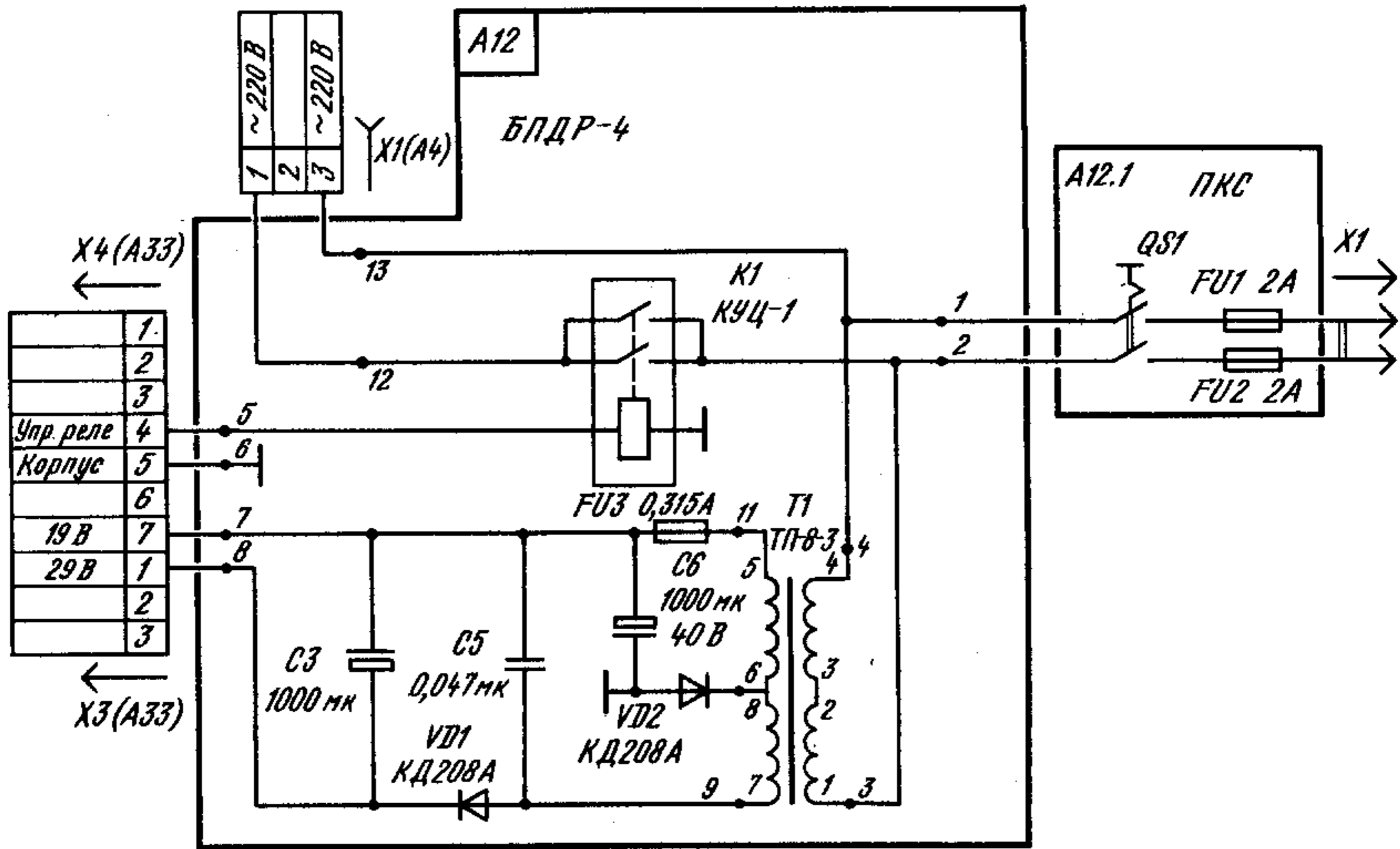
Принципиальная электрическая схема ПКС и БПДР-4
