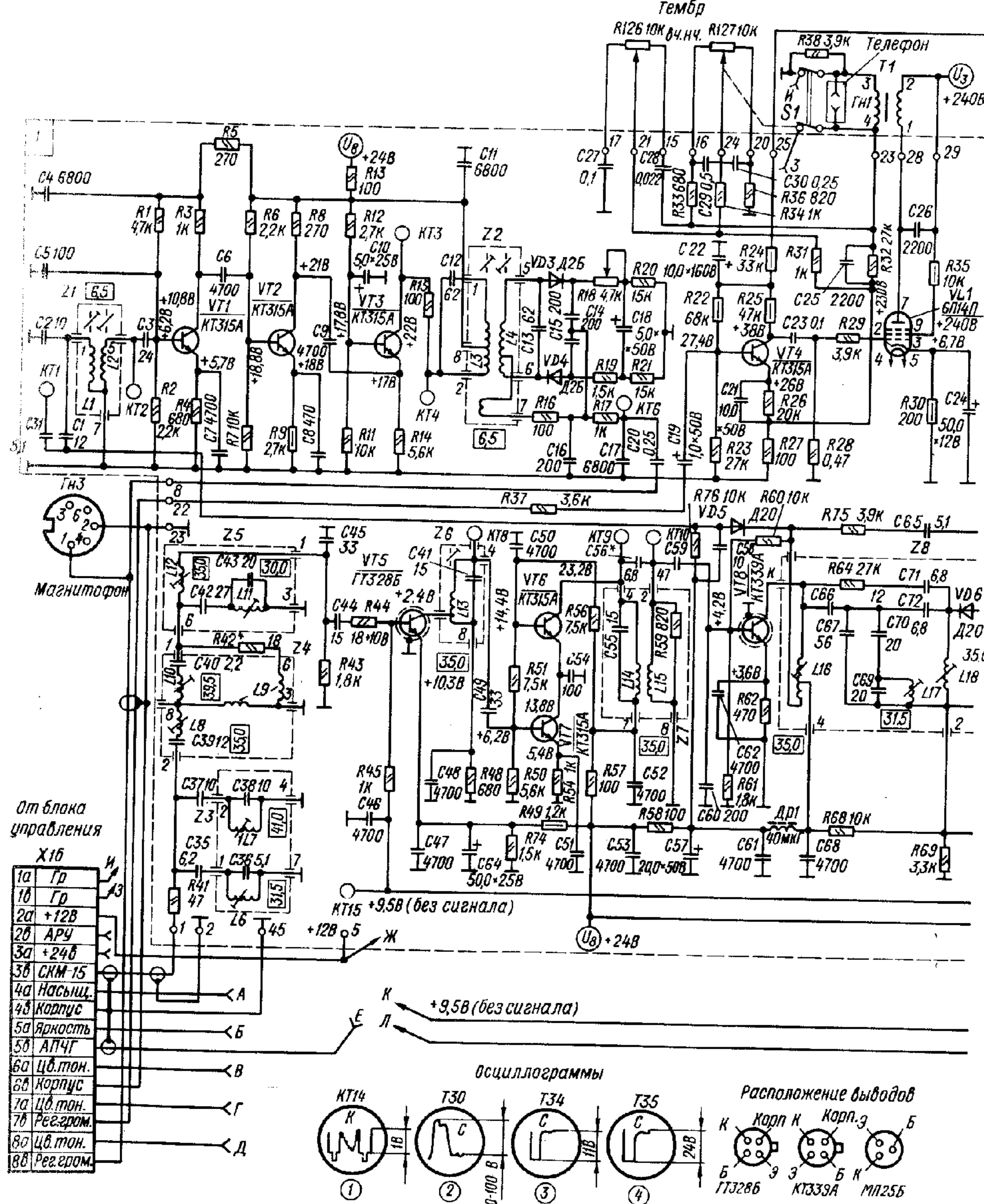
Принципиальная схема БРК-1 телевизора УЛПЦТ-59-И.
