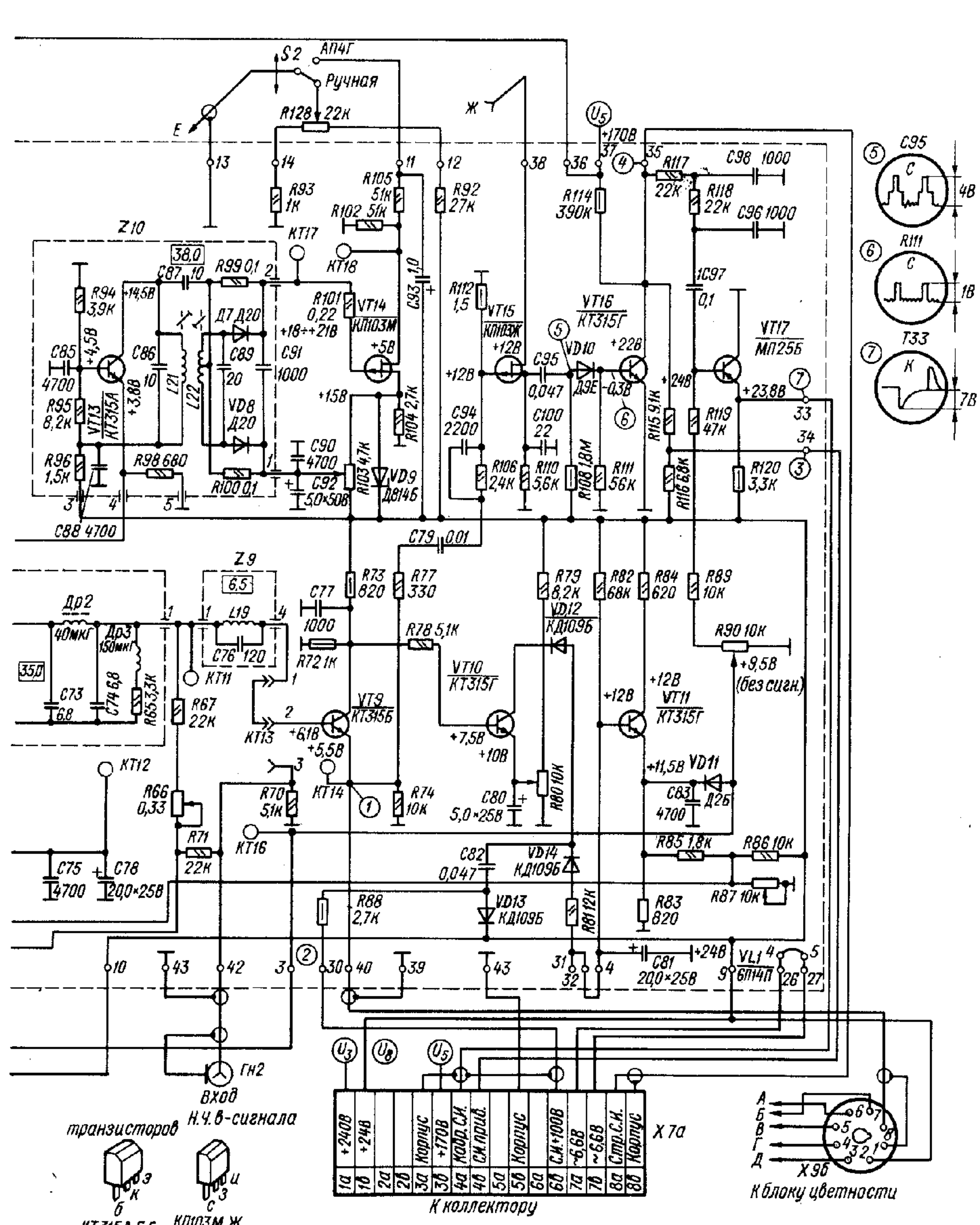
Принципиальная схема БРК-1 телевизора УЛПЦТ-59-И.
