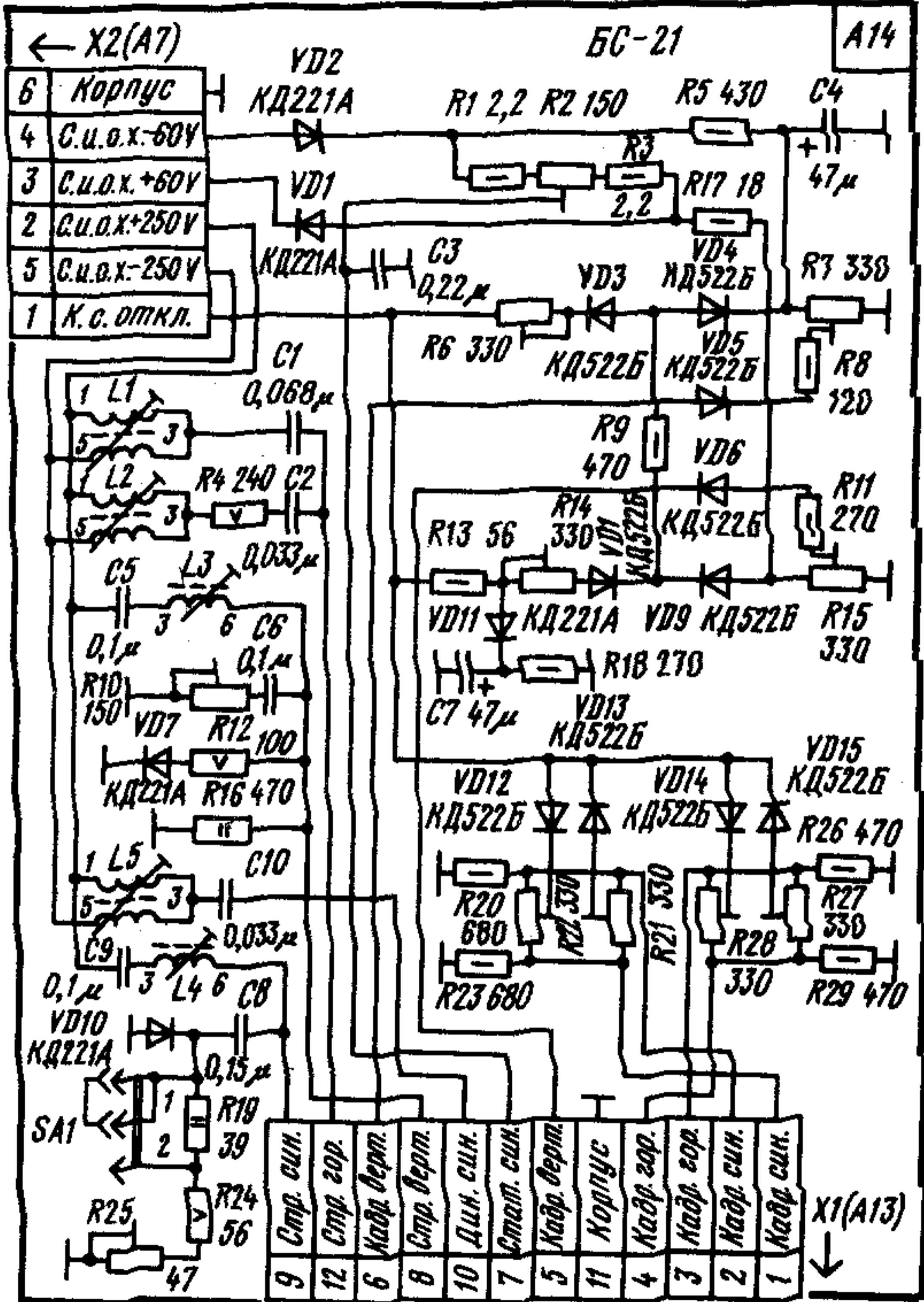
БС-21 Принципиальная схема блока сведения
