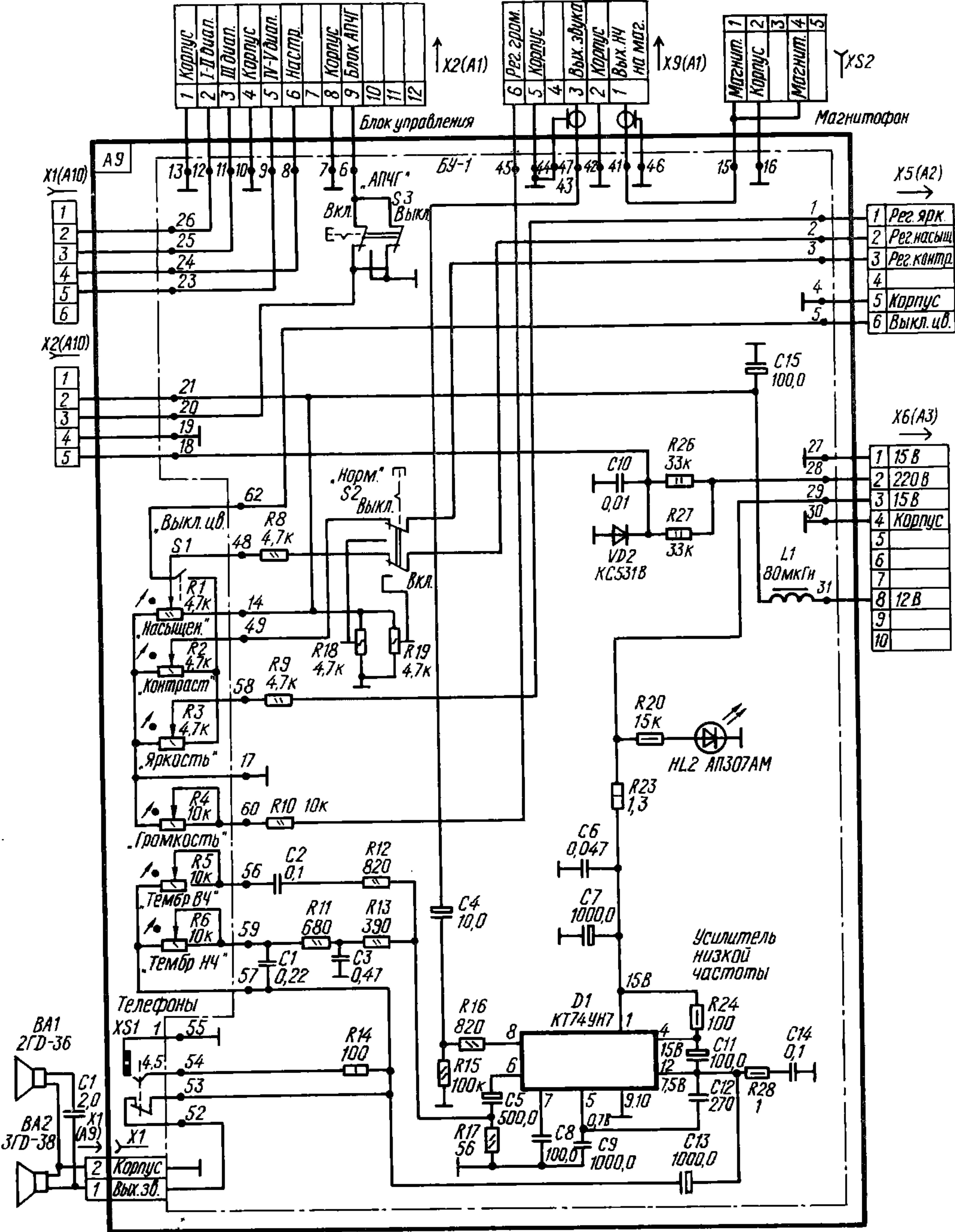
Рис. 4.44, б. Принципиальная схема блока управления А9.
