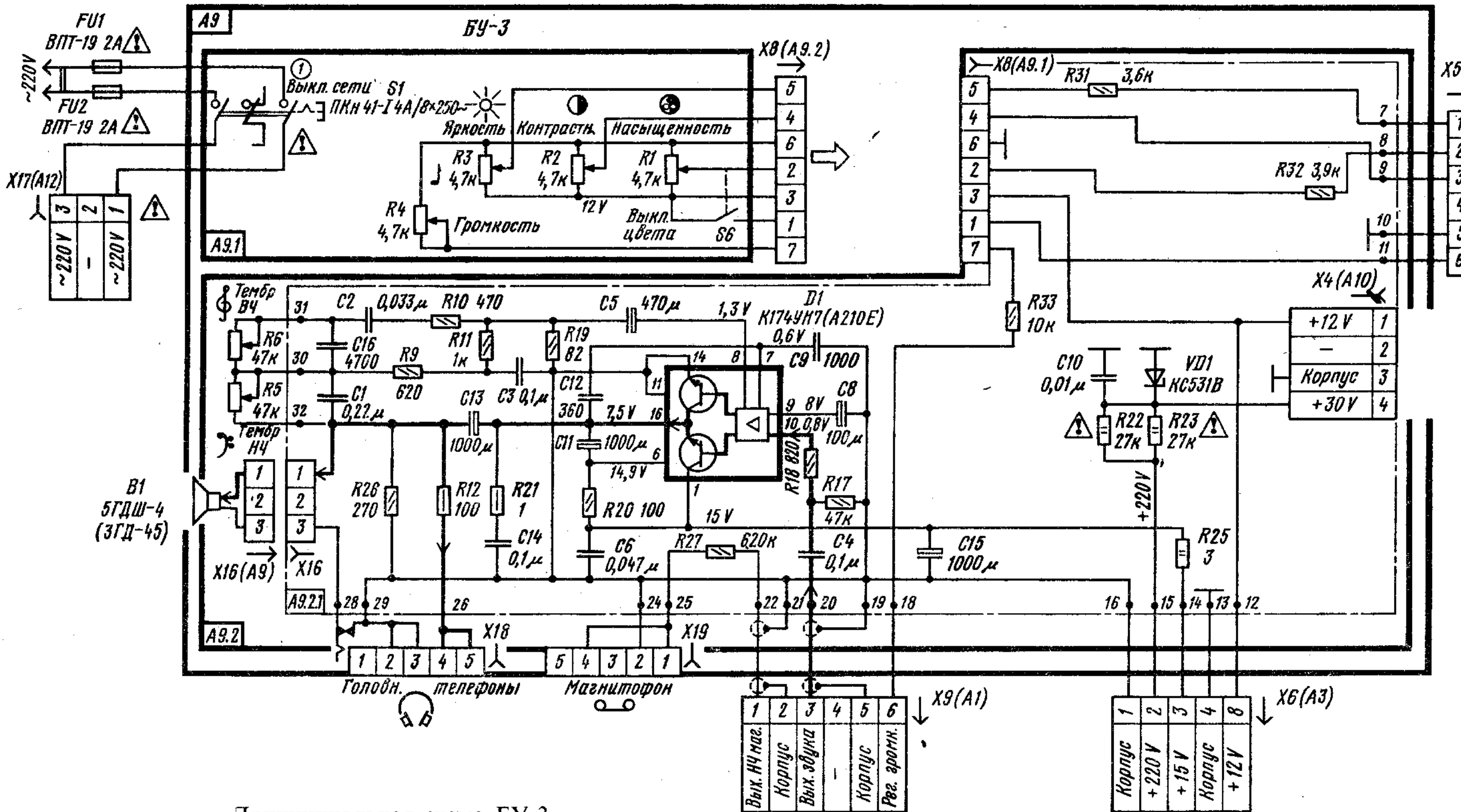
Принципиальная схема БУ-3
