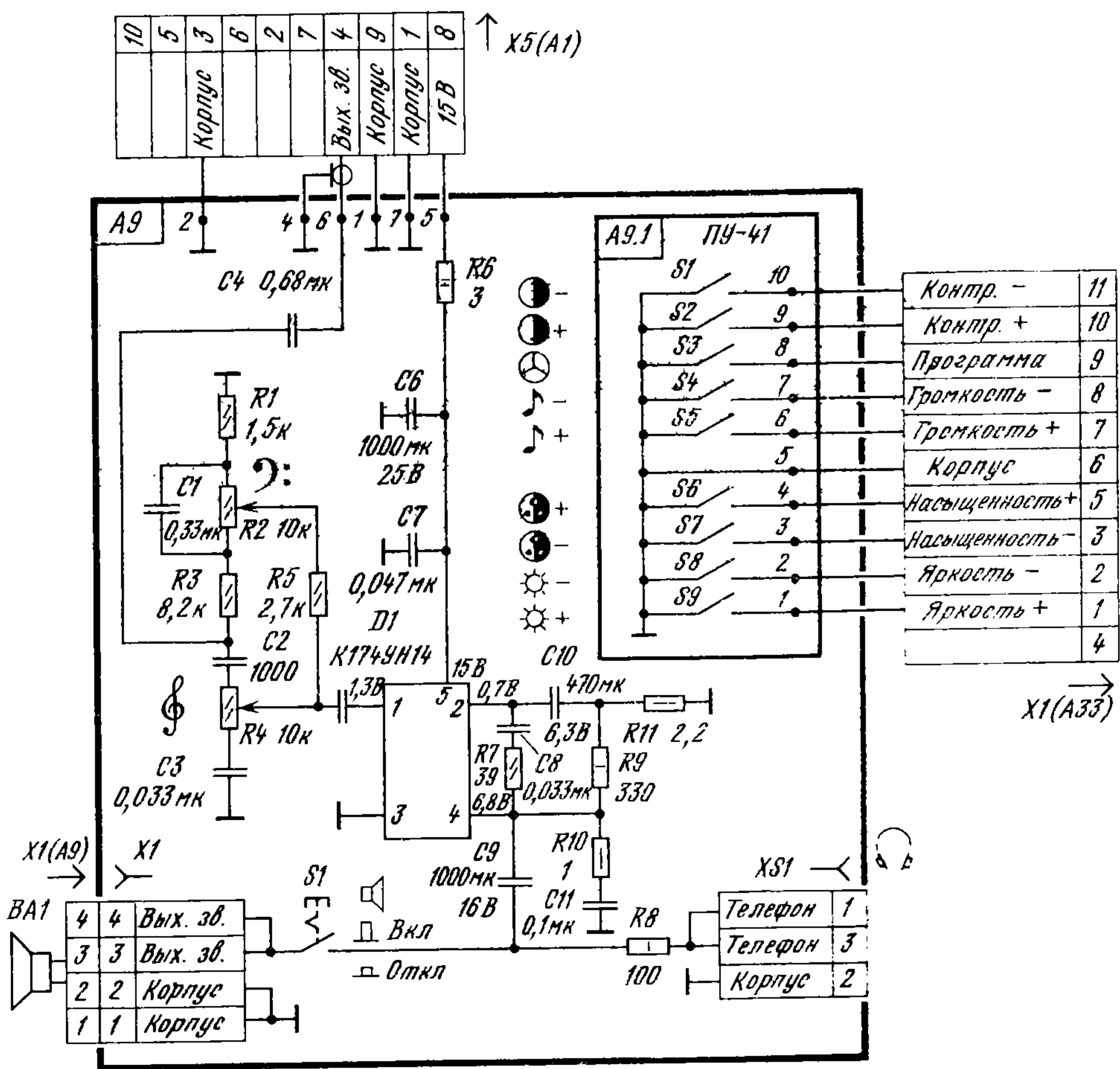
Принципиальная электрическая схема БУ-411
