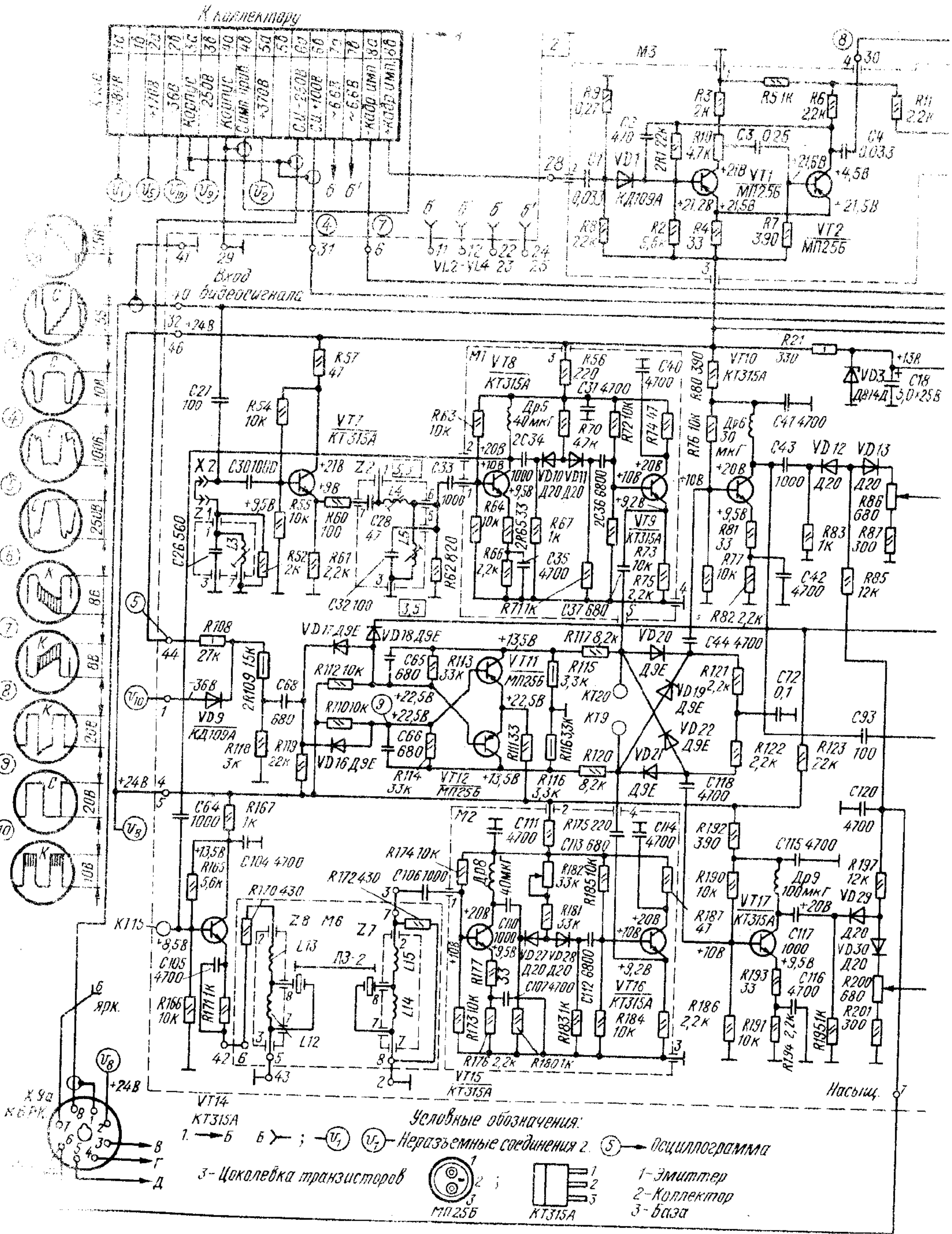
Принципиальная схема
