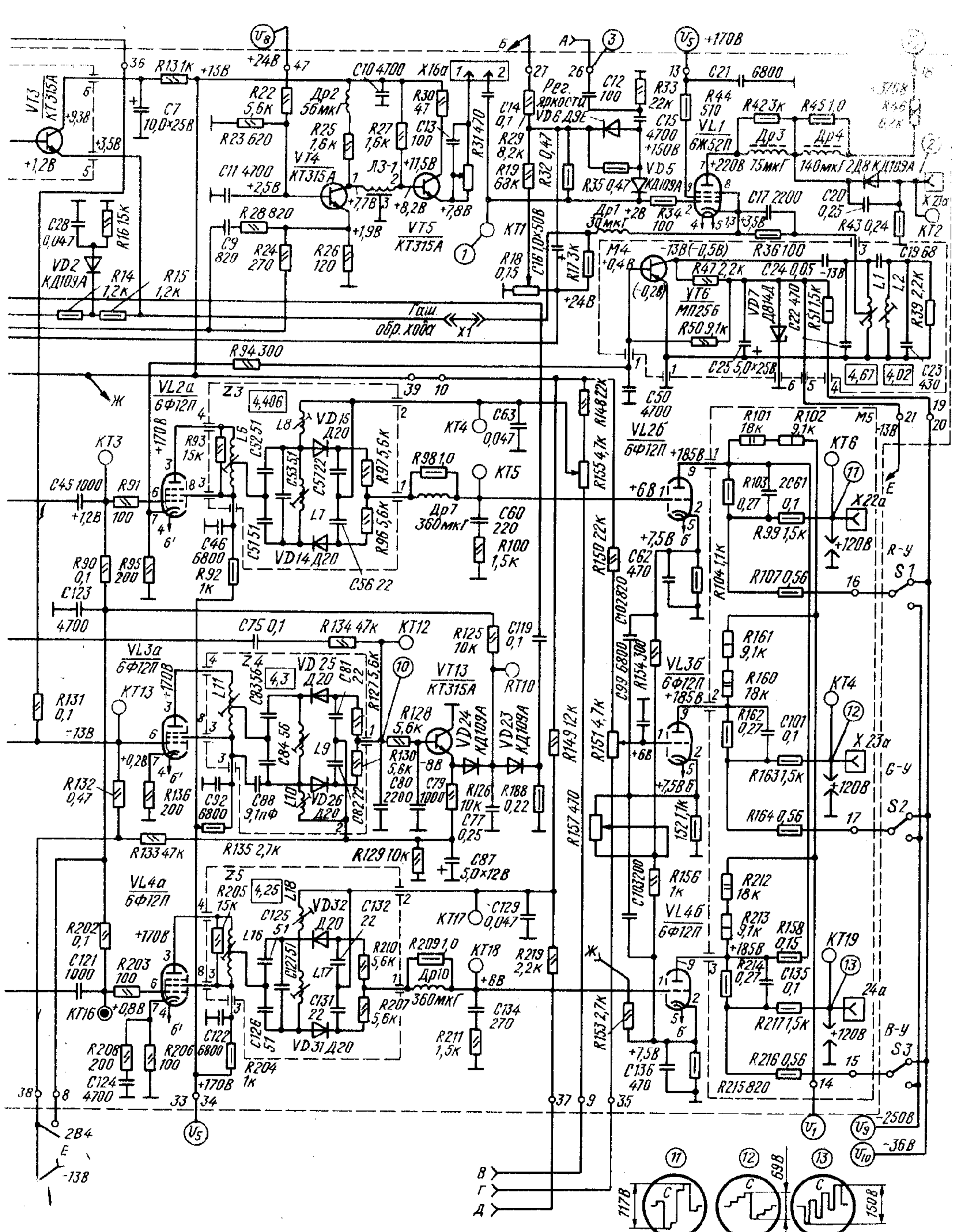
БЦ-1 телевизора УЛПЦТ-59-И.
