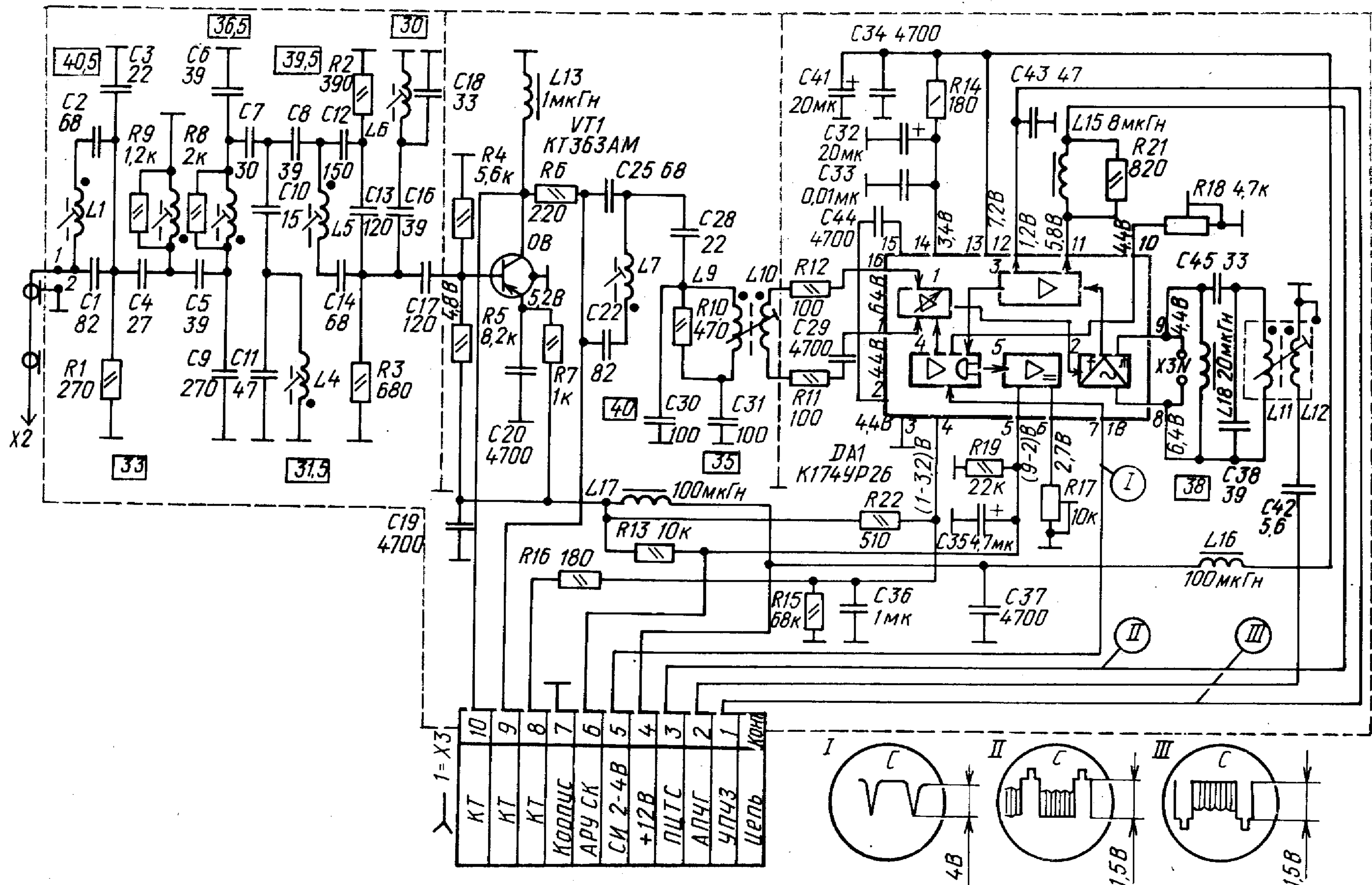
Электрическая принципиальная схема модуля УПЧИ УМ1-1
