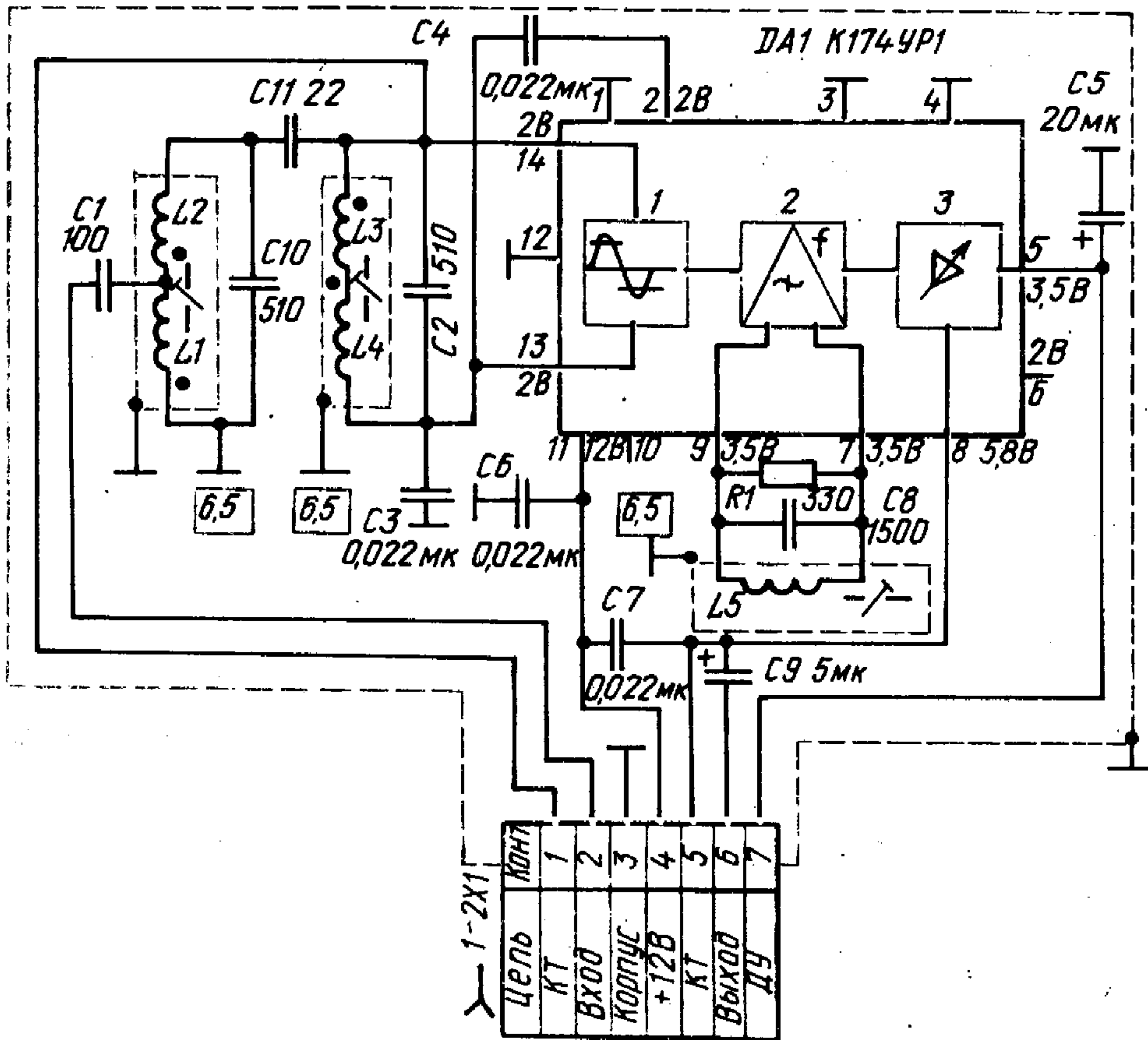
Электрическая принципиальная схема модуля УПЧЗ УМ1-2
