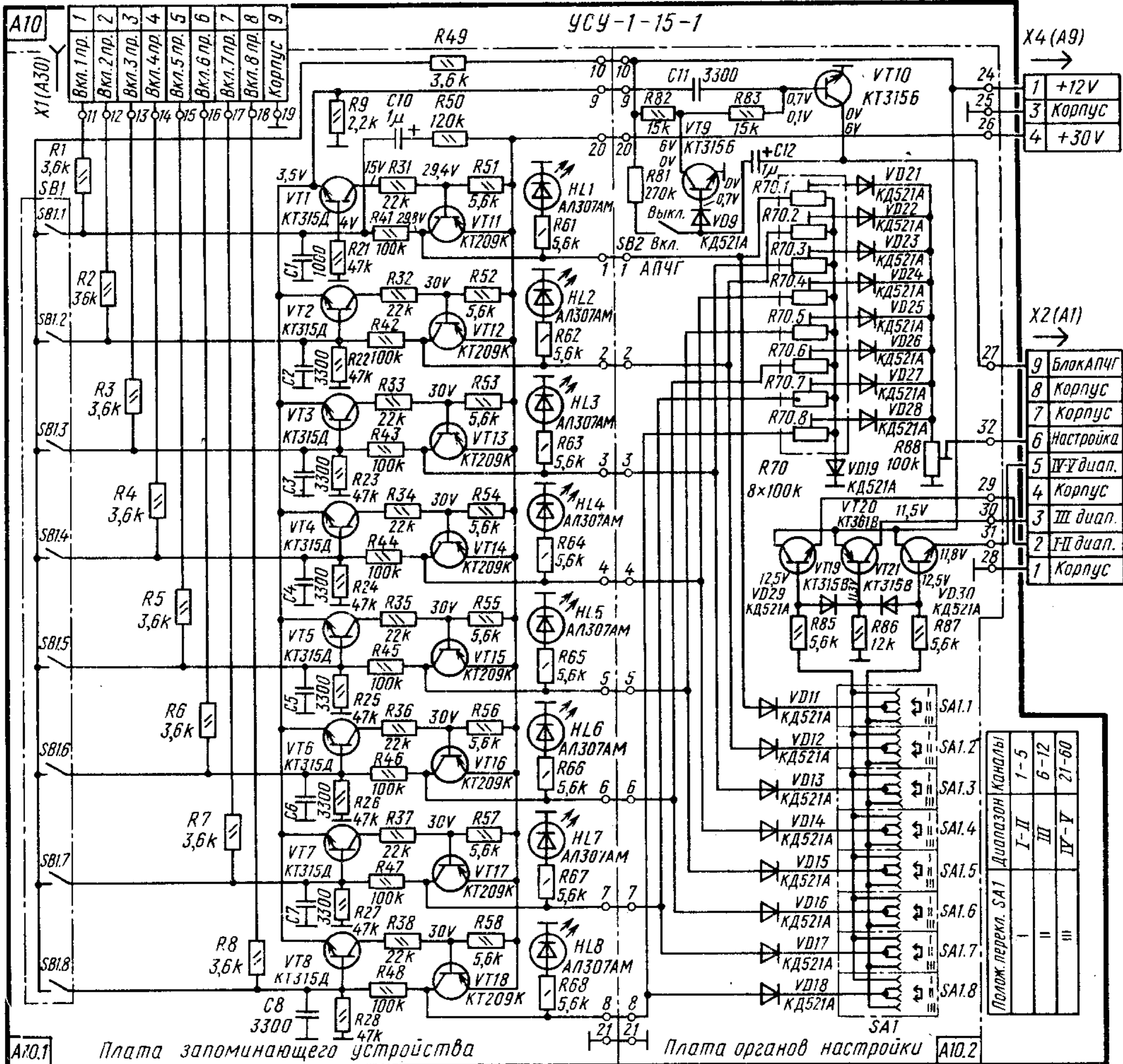
Принципиальная схема УСУ-1-15-1
