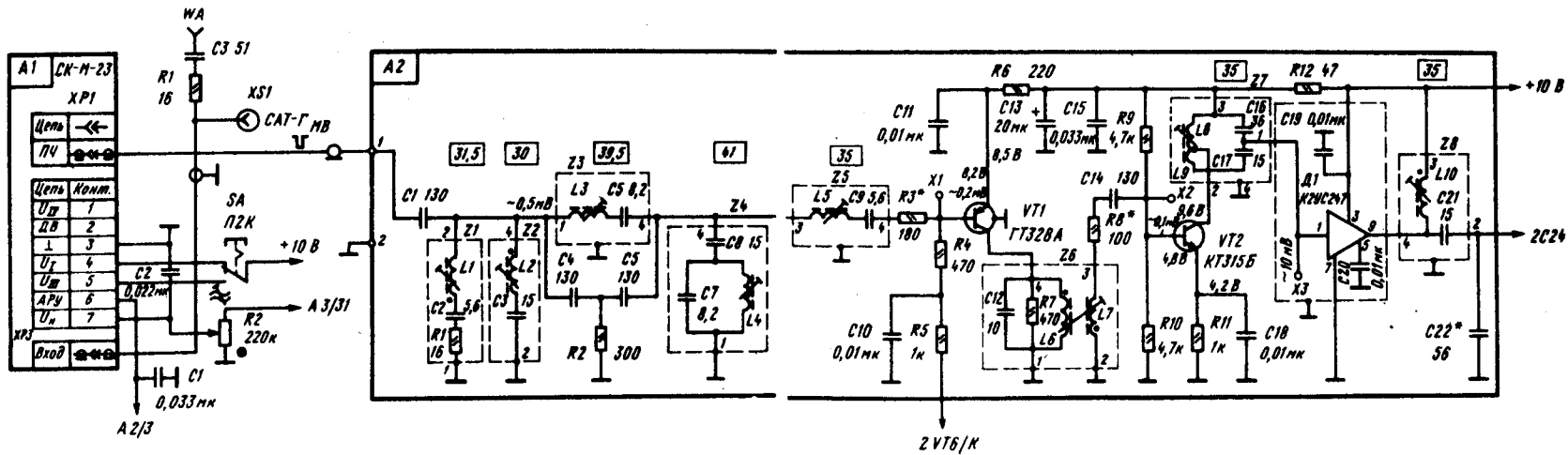
Принципиальная схема подключения СК и УПЧИ в телевизоре «Электроника-450»
