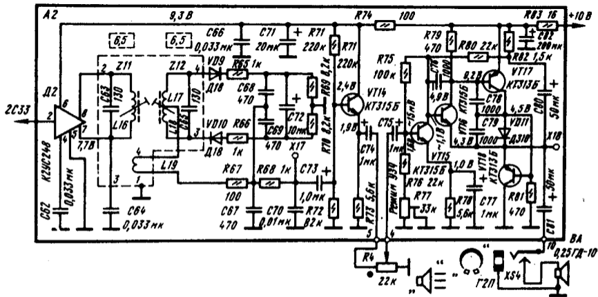
Принципиальная схема канала звука телевизора «Электроника-450»
