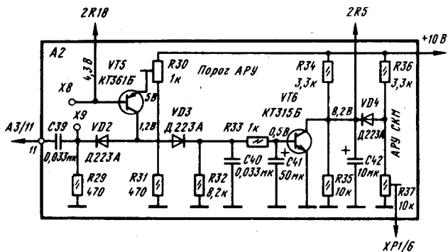
Принципиальная схема элементов АРУ телевизора «Электроника-450»
