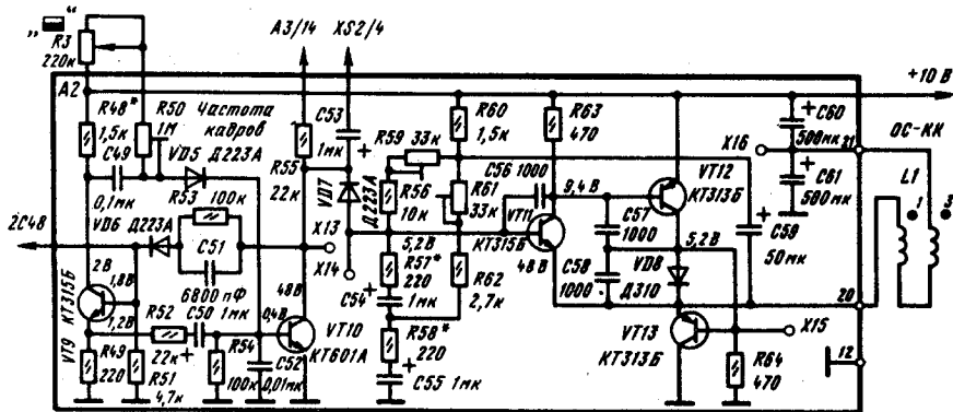
Принципиальная схема БКР телевизора «Электроника-450»
