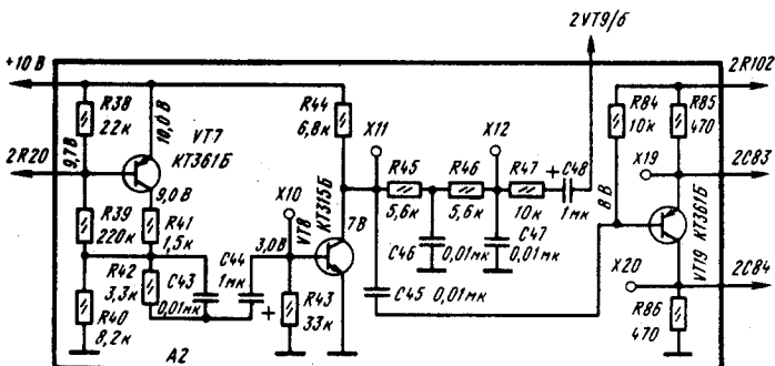
Принципиальная схема канала синхронизации телевизора «Электроника-450»
