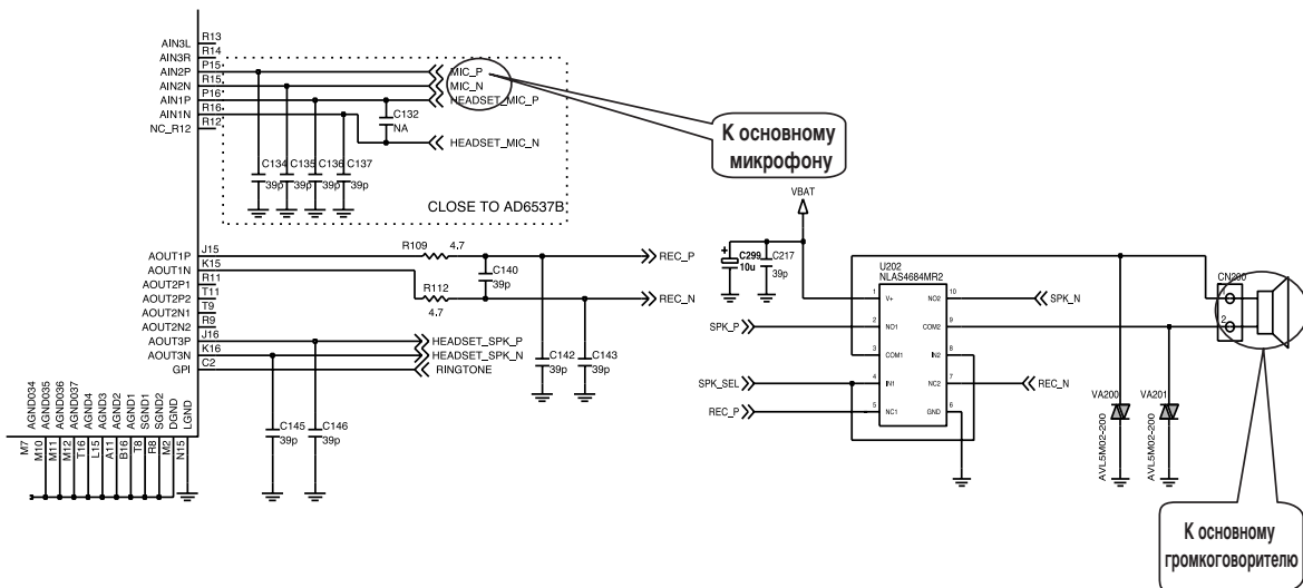
Рис. 3-20. Цепь динамика/микрофона модели B2150 (AD6537B)
