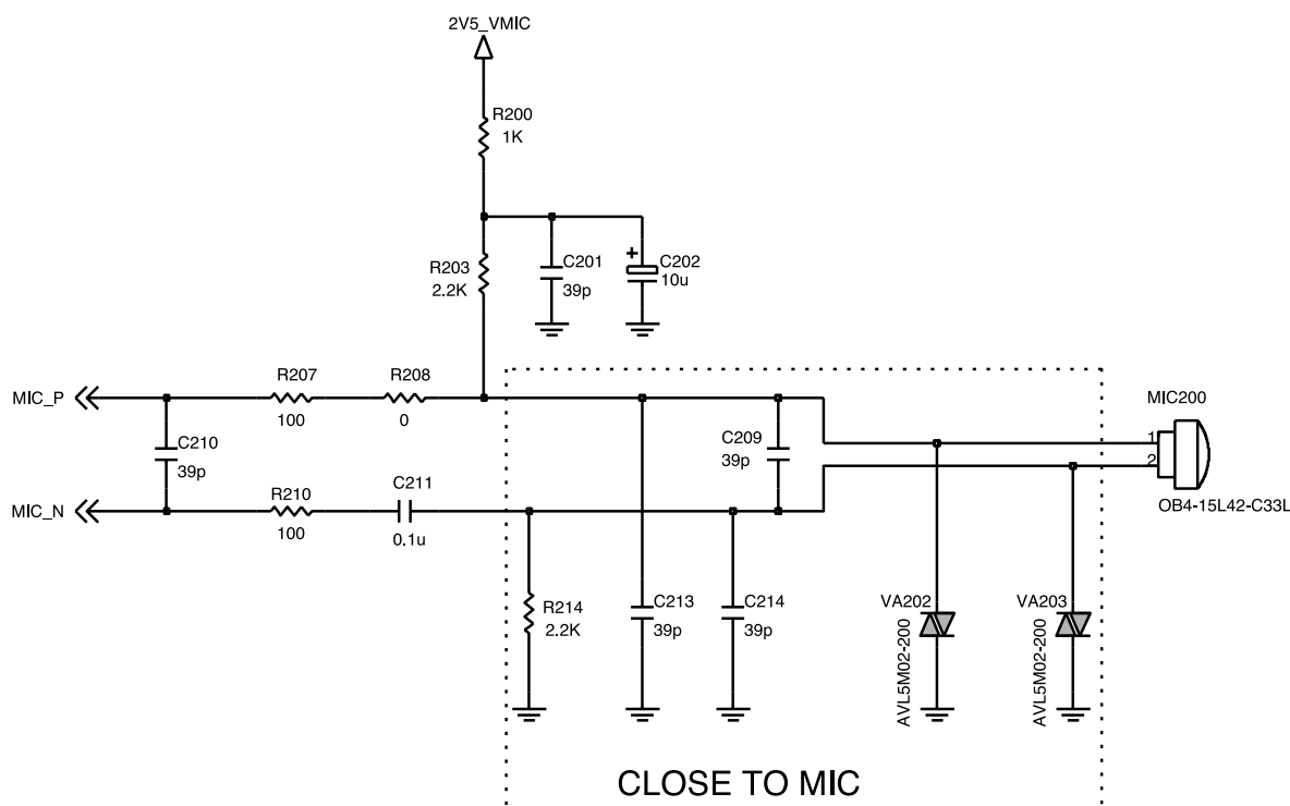
Рис. 3-28. Соединение микрофона с AD6537B
