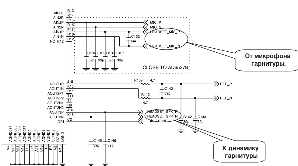
Рис. 3-19. Цепь динамика/микрофона гарнитуры модели B2150 (AD6537B)
