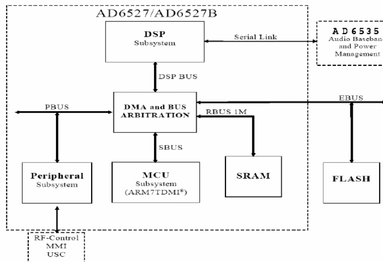
Рис. 3-10. Архитектура AD6527
